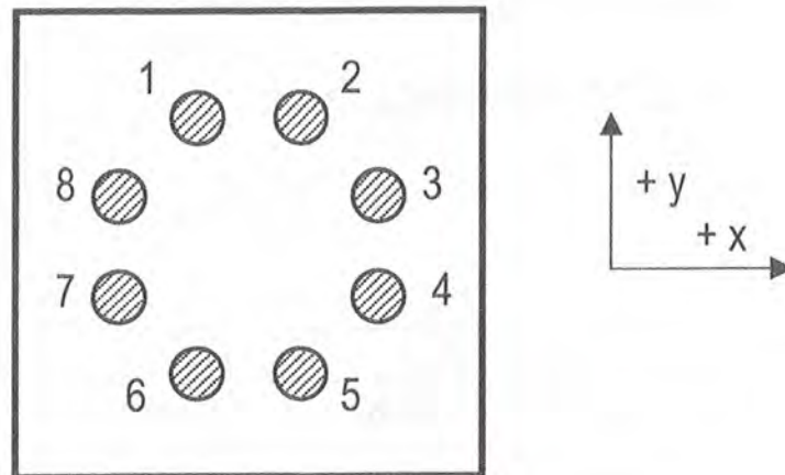
Achs-Randabstände der Anschlussbewehrung \varnothing 20 [ mm ]
